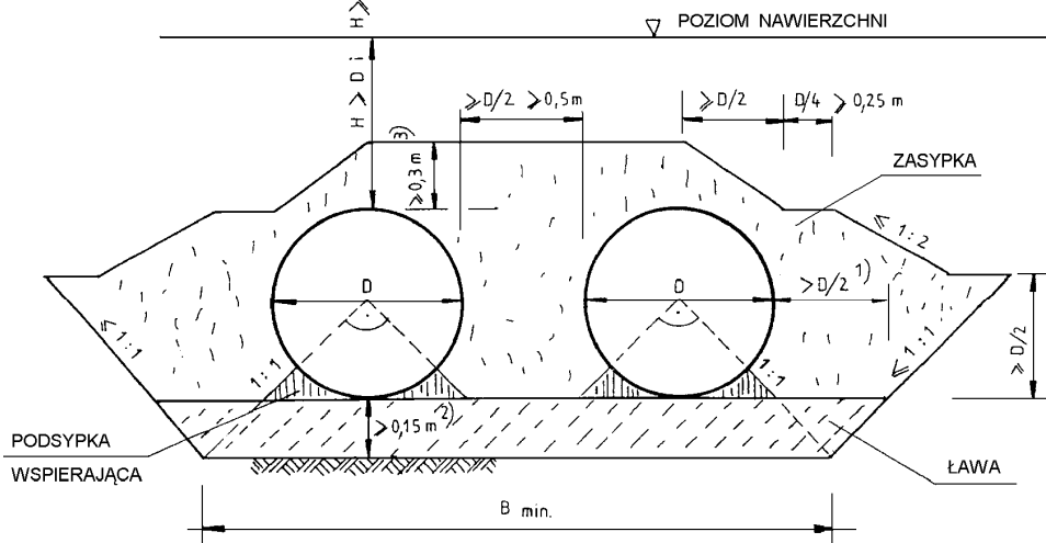
Rys. 9. Zasyпка nad przepustem dwururowym
