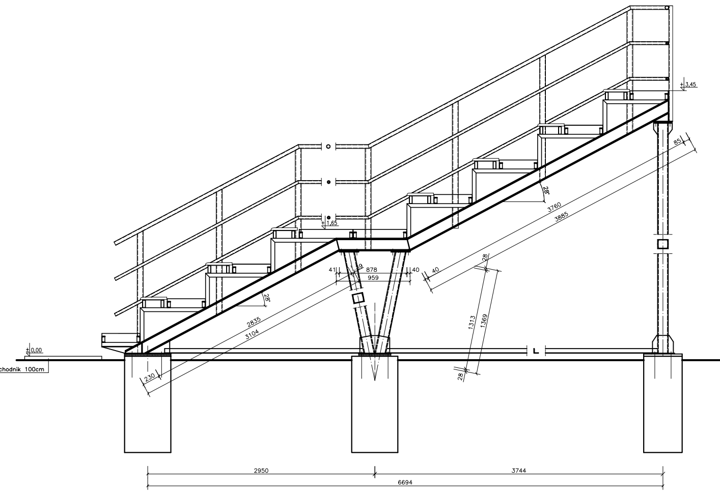
PRZEKRÓJ A-A
